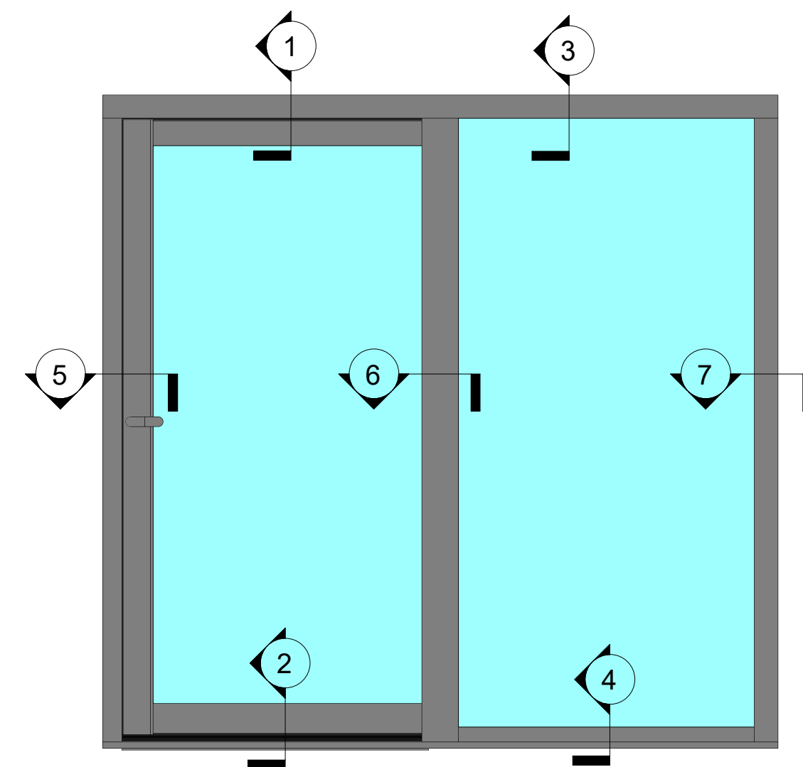
ELEVATION
