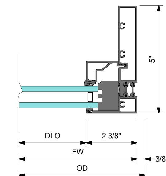
7 DETAIL 7 VERTICAL XO JAMB
